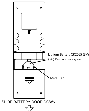
Abbildung 3. Austauschen der Batterie bei der Fernbedienung des MAC 310
